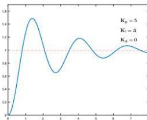
پاسخ سیستم با کنترلر PI
